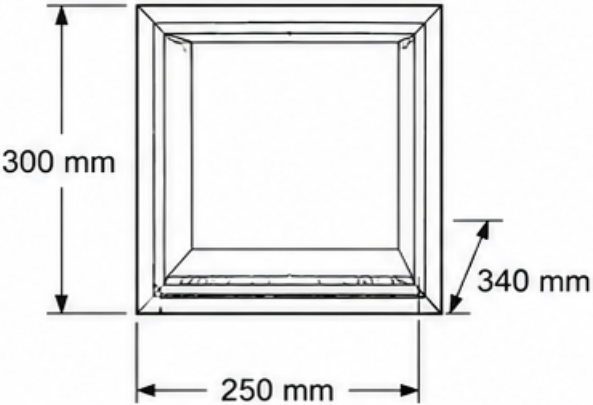
DIMENSIONS DU FOYER (HxLxP)
