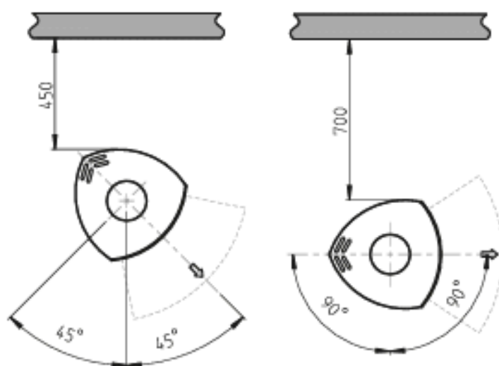
Afstand tot brandbare muur met draaibaar voetstuk
